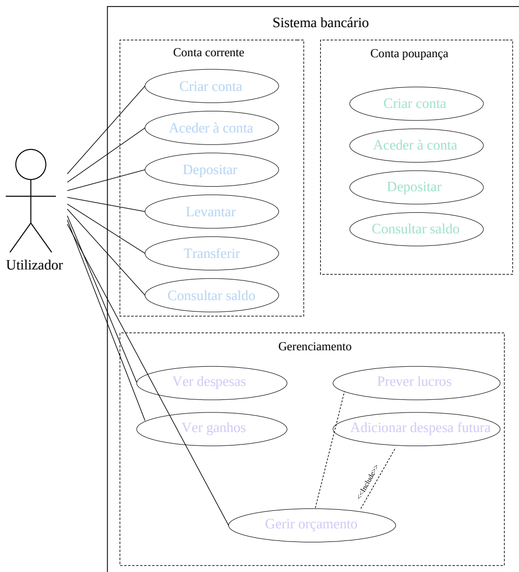
Figura 2 - Diagrama de Casos de Uso
