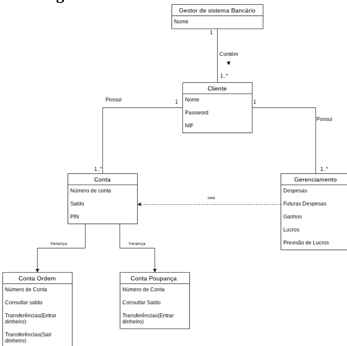
Figura 1 - Diagrama de Domínio
